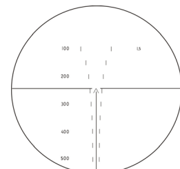
Сетка с дальномерной шкалой. Вид поля зрения.
