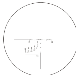
Сетка с дальномерной шкалой. Вид поля зрения.
