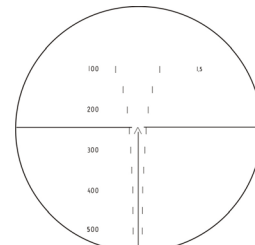
Сетка с дальномерной шкалой. Вид поля зрения.
